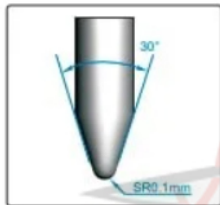
HS5D indenter
