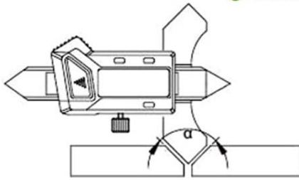
Groove Angle
